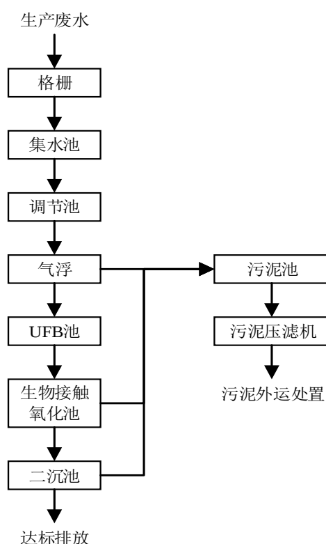
图 4-1 污水处理站污水处理工艺流程图
