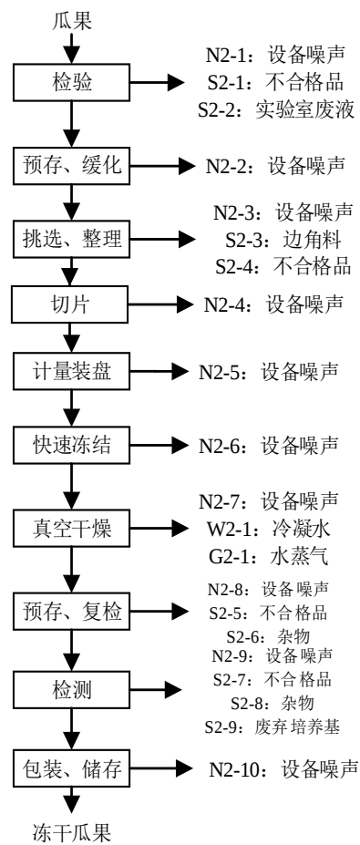
图 2-3 冻干瓜果生产工艺流程及产污环节图
