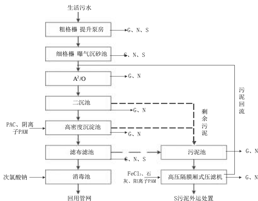
图 4-2 新滩生活污水处理厂工艺流程图
