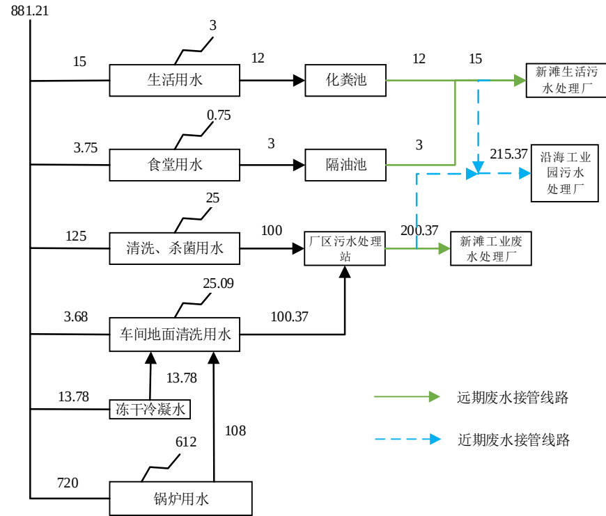
图2-1 项目用水量平衡图（单位：t/d）
