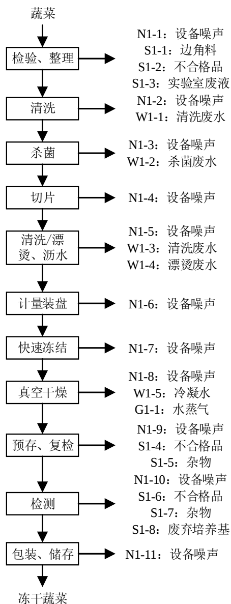
图 2-2 冻干蔬菜生产工艺流程及产污环节图
