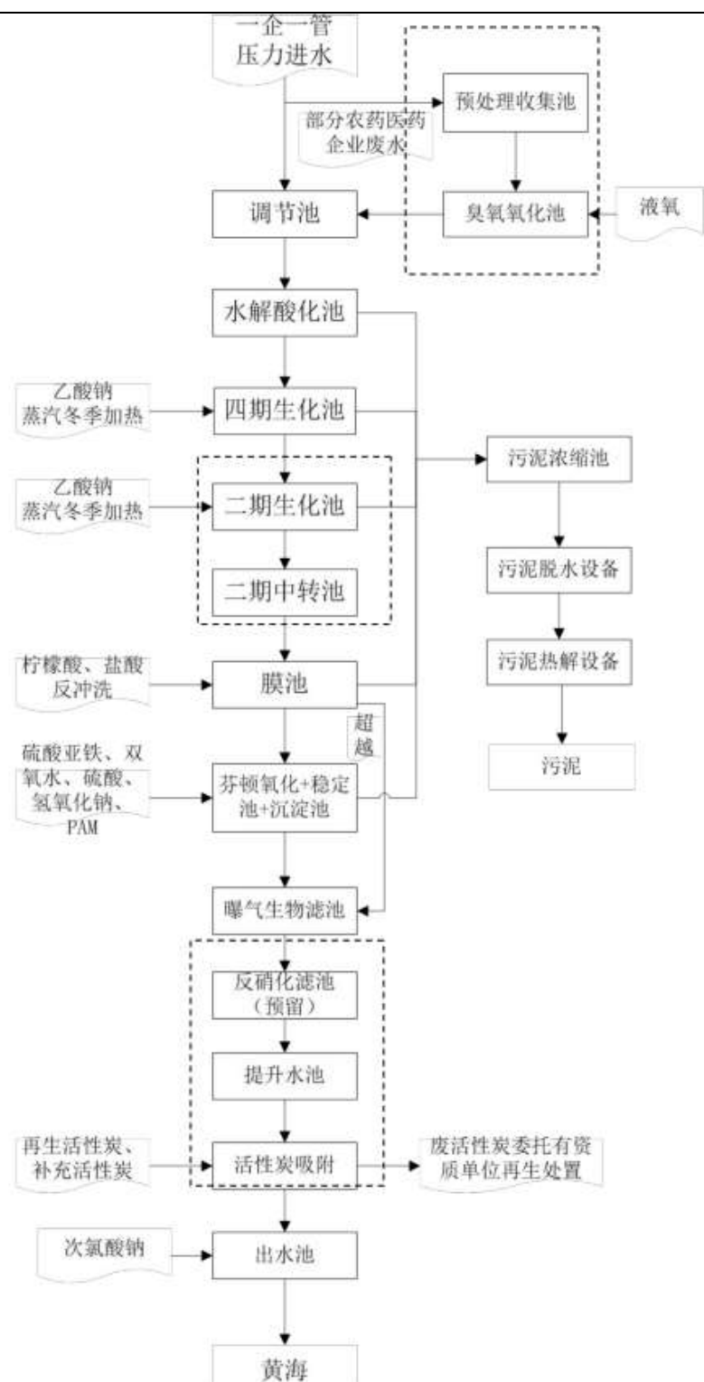
图 4-4 沿海工业园污水处理厂处理工艺流程图
