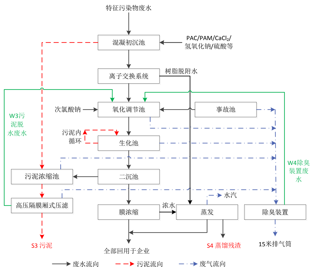
图 4-3 新滩工业污水处理厂二期工艺流程图
