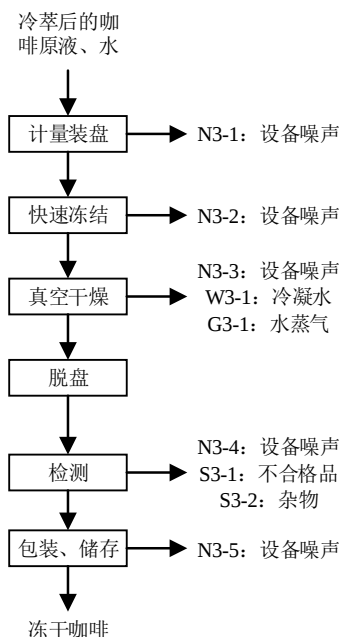
图2-4 冻干咖啡生产工艺流程及产污环节图
